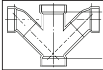
Combinaison double WYE / 1 / 8 courbure
