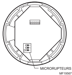
Fig. 8. Microrupteurs.
