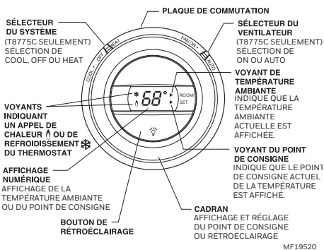
Fig. 10. Thermostat T8775 (caractéristiques et fonctionnement).
