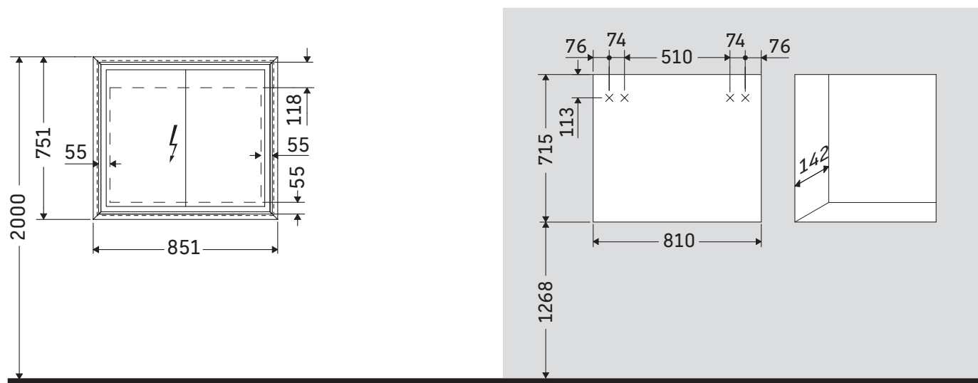
Ausschnittgröße für Einbauschränke
