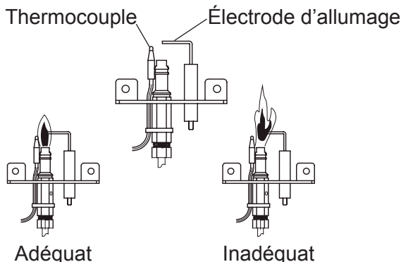
FIGURE 4 Flamme appropriée de la veilleuse
