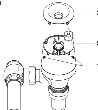
Fig. 11a BATERÍA ESTÁNDAR
