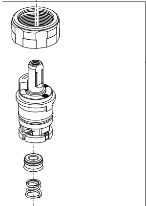
RP101504 Stem Unit Assembly, Seat & Spring, Bonnet Nut Ensamble de la Unidad del Vástago, Asiento y Resorte, Bonete Obturateur, siège et ressort, écrou à chapeau
