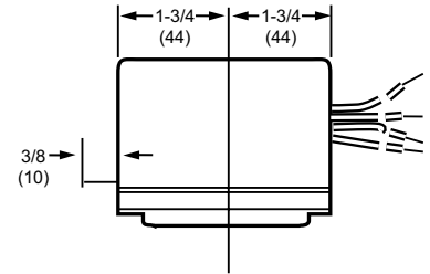
VU5 ACTUATOR
