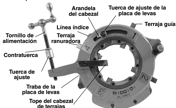
Figura 1 – Cabezal de terrajas ranuradoras 725
