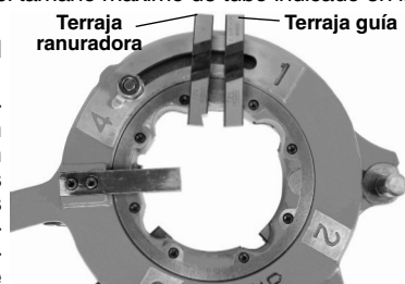
Figura 2 – Colocación de las terrajas
